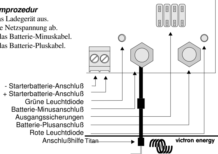
Abbildung 3. Lage der Batterie- Anschlüsse
