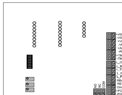
Abbildung 7. Lage des DIP-schalters und der Potentiometer
